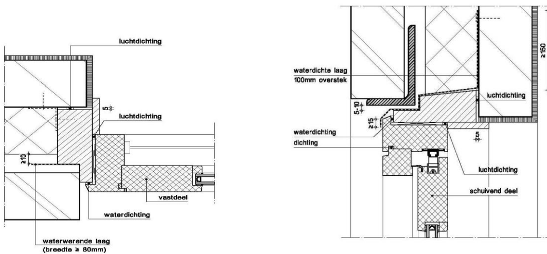
Horizontale doorsnede
